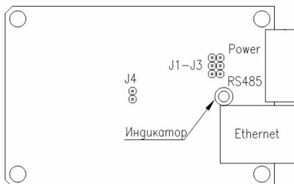
Рисунок 2 - Расположение перемычек на плате
