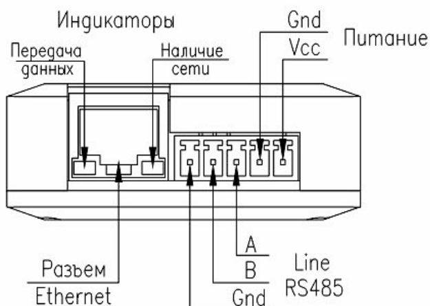
Рисунок 1 - Подключение устройства и индикация режимов работы
