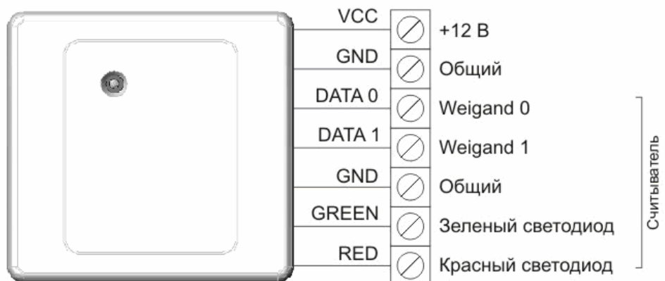
Рис. 2. Подключение по интерфейсу Weigand
