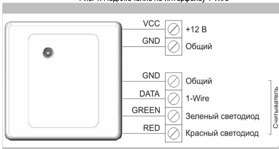
Рис. 1. Подключение по интерфейсу 1-Wire
