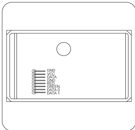
Рисунок 1 - Подключение по интерфейсу 1-Wire
