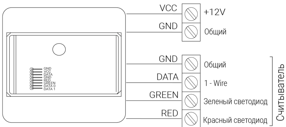
Рисунок 1 - Подключение по интерфейсу 1-Wire
