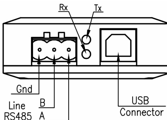
Рисунок 1 - Подключение устройства и индикация режимов работы
