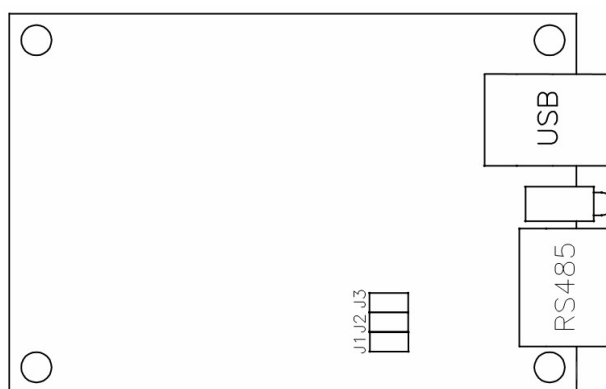
Рисунок 2 - Расположение перемычек на плате
