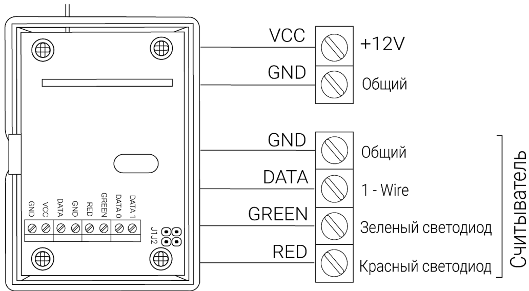
Рисунок 1 - Подключение по интерфейсу 1-Wire
