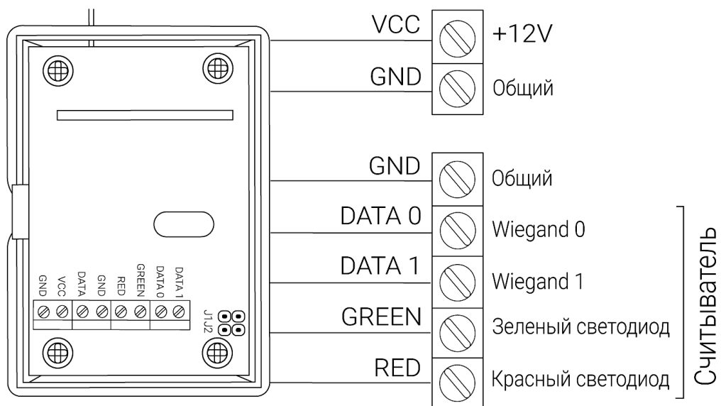
Рисунок 2 - Подключение по интерфейсу Wiegand 26
