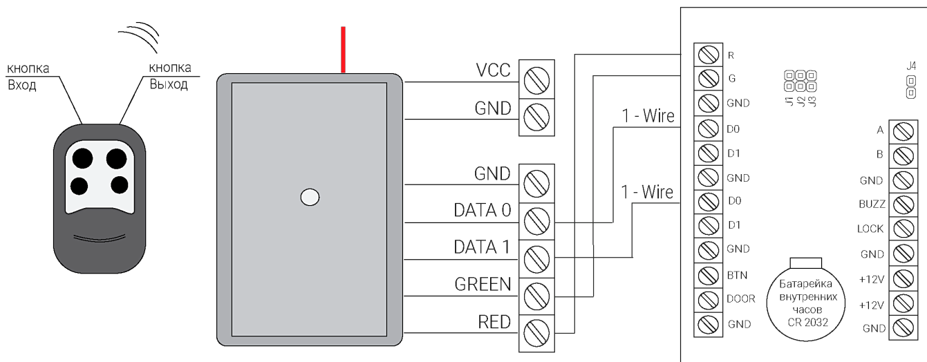
Рисунок 3 - Схема подключения считывателя радио брелоков для работы одной точки прохода на «Вход» и «Выход»
